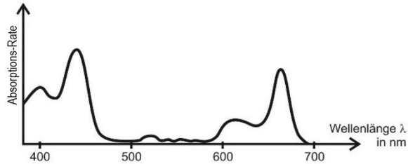
Absorptionsspektrum von Chlorophyll a
